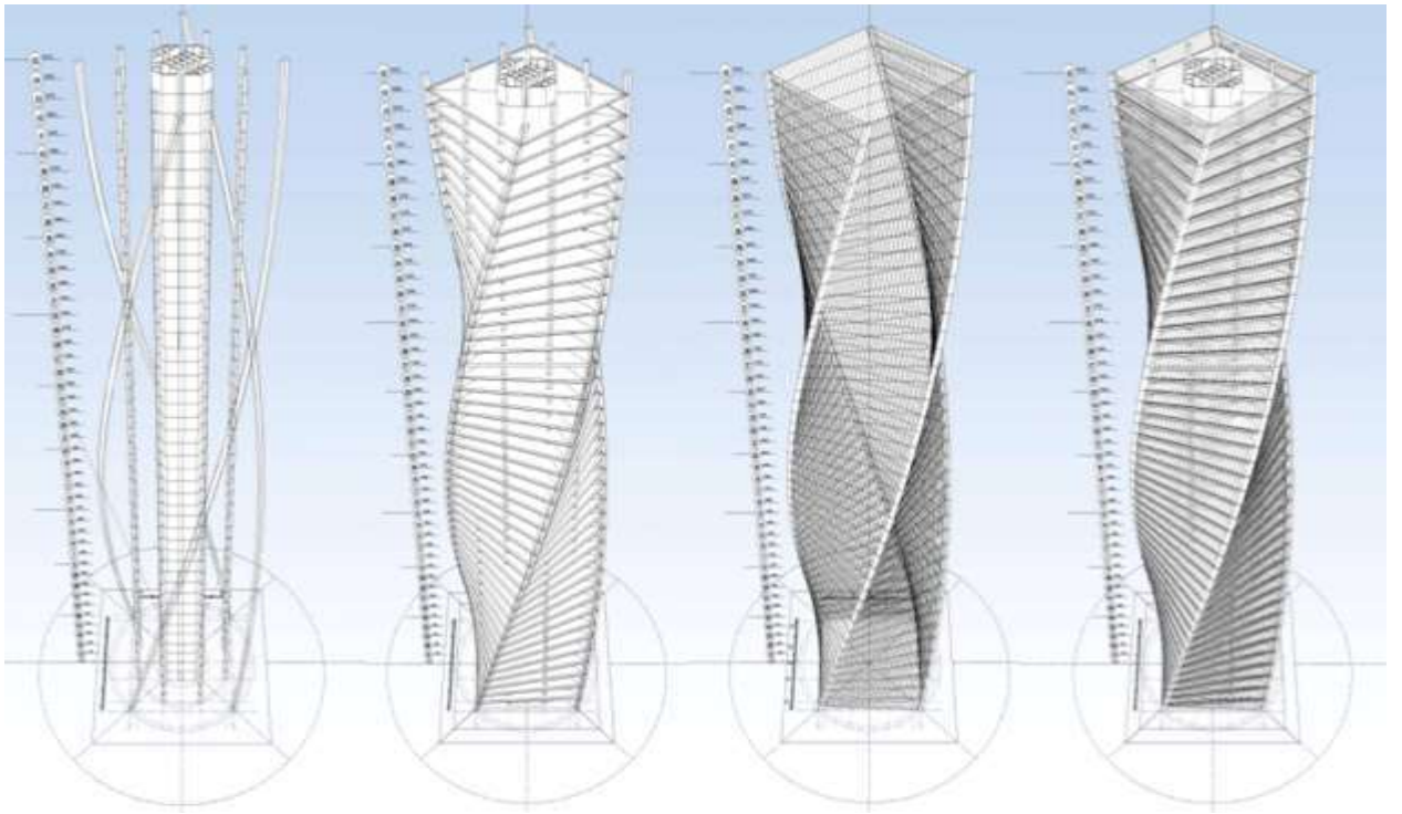
Рис. 2. Проект башни «Эволюция»
