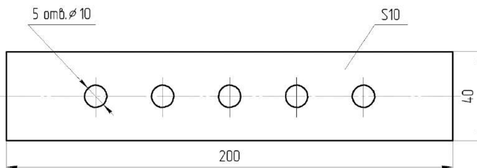
Рисунок 2. Верхняя деталь
